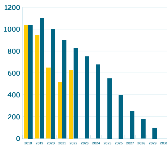
Bränsletransporter och -hantering, ton CO 2 e
