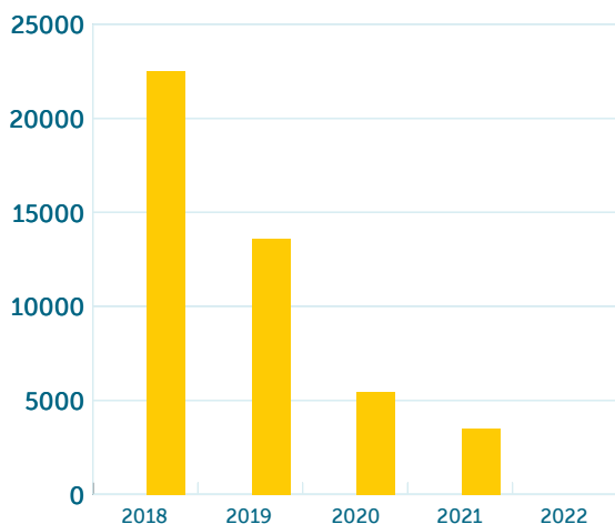
Koldioxid från torveldning, ton CO 2 e
