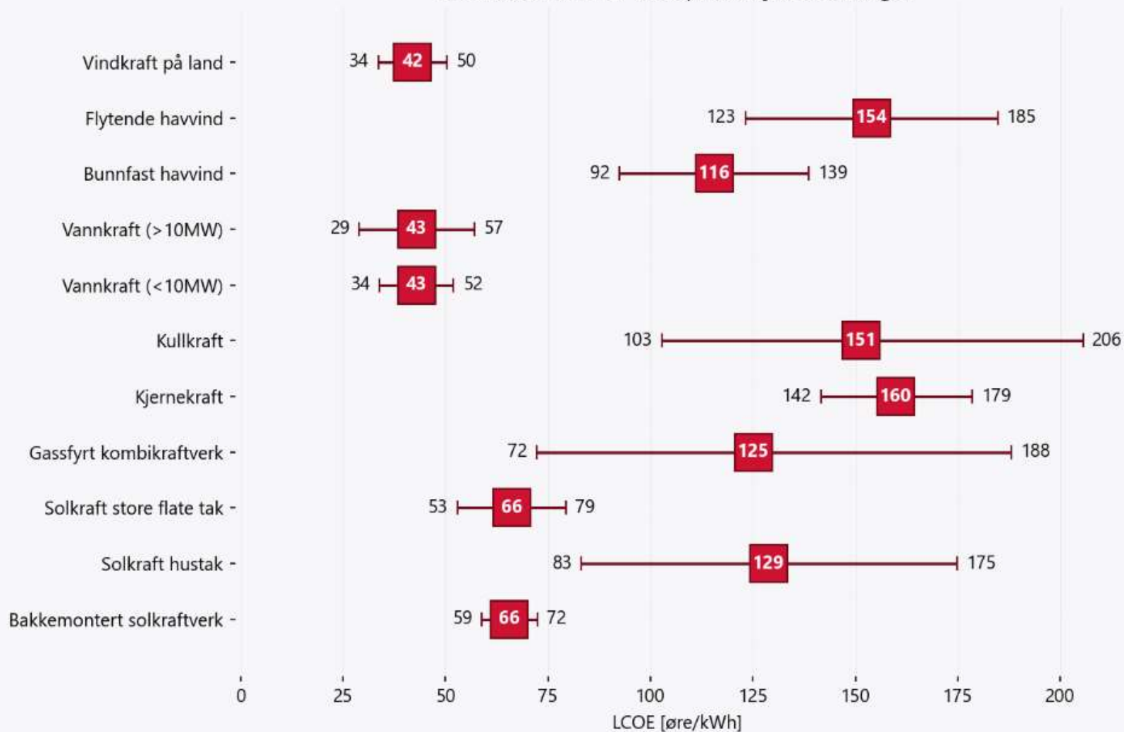
LCOE [øre/kWh] for ulike produksjonsteknologier
